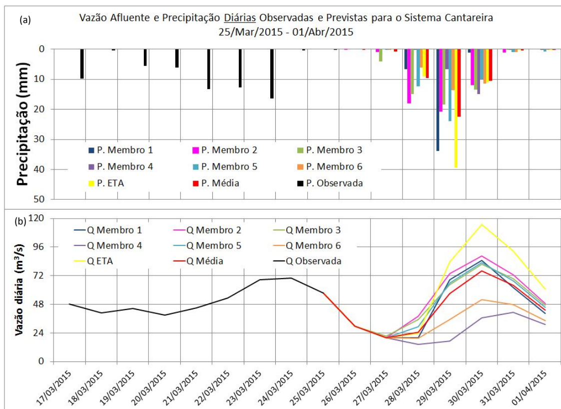
Figura 9. (a) Corresponde às precipitações diárias observadas (P.Observada, barra preta), as previsões do ETA/CPTEC/INPE 40km (6 membros), do ETA/CPTEC/INPE 15km e a média das previsões (barra vermelha). A linha preta apresenta as vazões diárias (Q) observadas, as demais linhas apresentam as vazões previstas a partir das diferentes previsões de precipitação.
