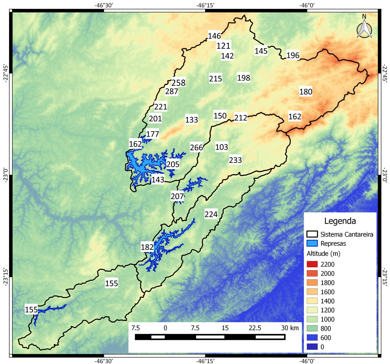
Figura 5. Precipitação observada acumulada (em mm) de 01 a 25 de março nos pluviômetros do CEMADEN e DAEE/SAISP nas sub-bacias de captação do Sistema Cantareira (contornos em preto). As cores representam alturas topográficas com relação ao nível do mar de acordo com a escala da direita.
