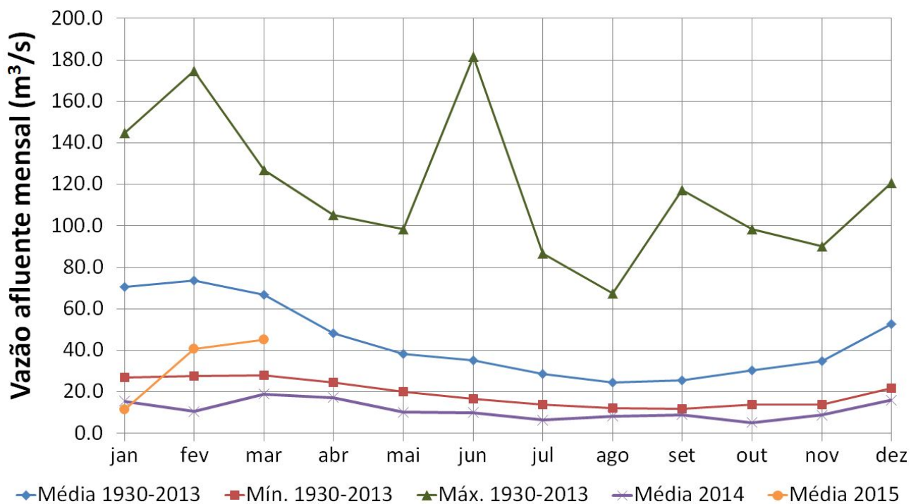
Figura 2. Vazão afluente (em m^3/s ) do Sistema Cantareira (Sistema Equivalente + Paiva Castro). A linha laranja refere-se à vazão média mensal até 25 de março de 2015 e a roxa à vazão média mensal de 2014. A linha em azul corresponde às vazões médias mensais para o período 1930 – 2013. As linhas verde e vermelha referem-se, respectivamente, aos máximos e mínimos absolutos da série histórica mensal no período 1930 – 2013.
