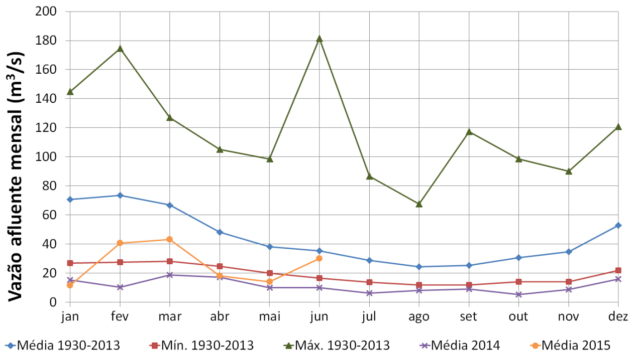
Figura 2. Vazão afluente (em m^3/s ) do Sistema Cantareira (Sistema Equivalente + Paiva Castro). A linha laranja refere-se à vazão média mensal até 03 de junho de 2015 e a roxa à vazão média mensal de 2014. A linha em azul corresponde às vazões médias mensais para o período 1930 – 2013. As linhas verde e vermelha referem-se, respectivamente, aos máximos e mínimos absolutos da série histórica mensal no período 1930 – 2013.
