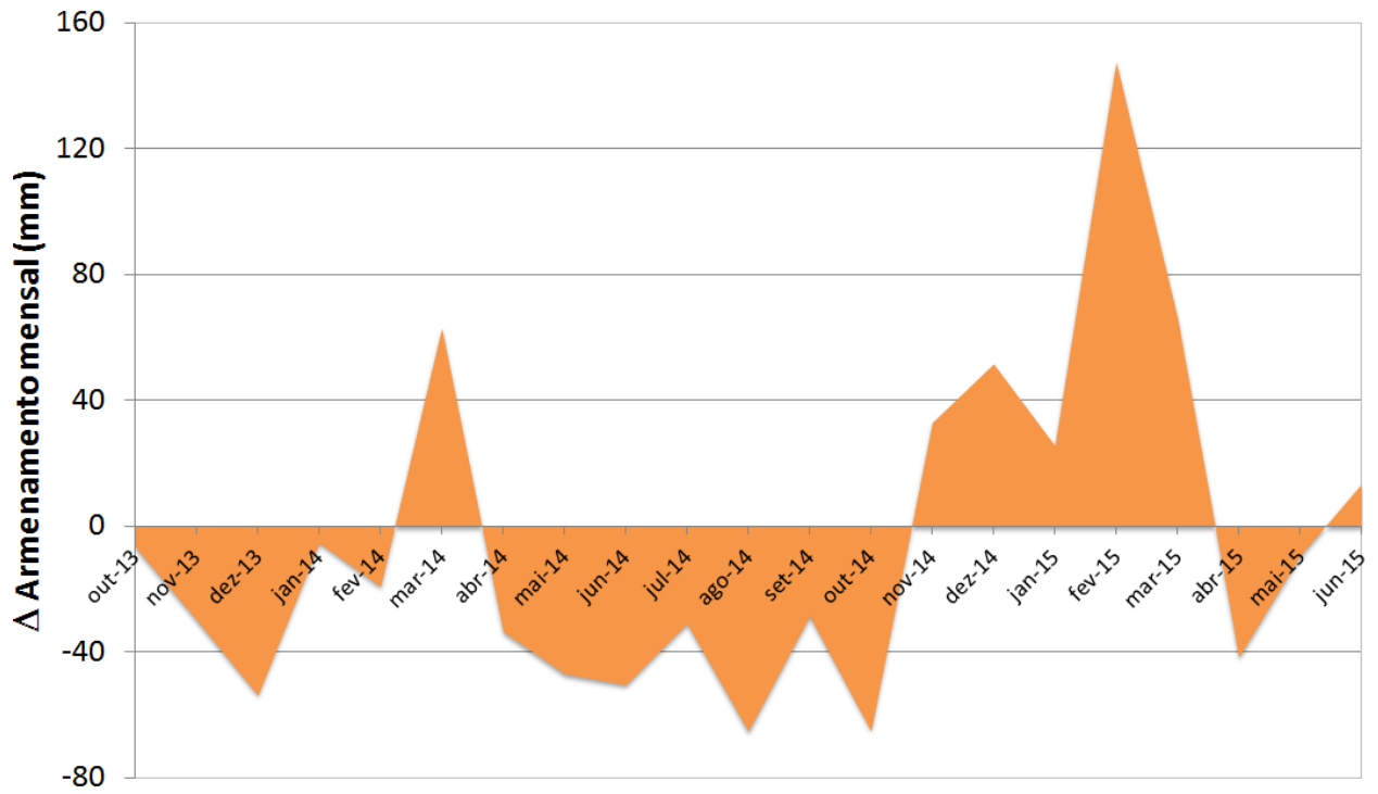
Figura 3. Variação média mensal do armazenamento de água no solo (em mm) para as sub-bacias do Sistema Cantareira). O valores negativos indicam déficit de água no solo.
