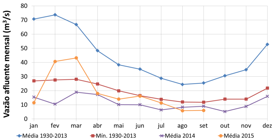
Figura 2. Vazão afluente (em m^3/s ) do Sistema Cantareira (Sistema Equivalente + Paiva Castro). A linha laranja refere-se à vazão média mensal até 02 de setembro de 2015 e a roxa à vazão média mensal de 2014. As linhas em azul e vermelho correspondem, respectivamente, às vazões médias mensais para o período 1930 – 2013 e aos mínimos absolutos da série histórica mensal no período 1930 – 2013.
