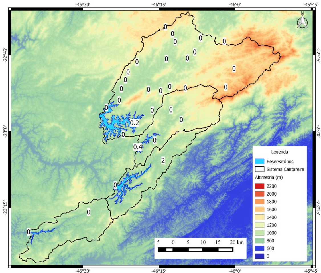
Figura 4. Precipitação observada acumulada (em mm) nos pluviômetros do CEMADEN e DAEE/SAISP nas sub-bacias de captação do Sistema Cantareira (contornos em preto). As cores representam alturas topográficas com relação ao nível do mar de acordo com a escala da direita.
