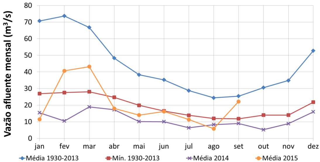
Figura 2. Vazão afluente (em m^3/s ) do Sistema Cantareira (Sistema Equivalente + Paiva Castro). A linha laranja refere-se à vazão média mensal até 16 de setembro de 2015 e a roxa à vazão média mensal de 2014. As linhas em azul e vermelho correspondem, respectivamente, às vazões médias mensais para o período 1930 – 2013 e aos mínimos absolutos da série histórica mensal no período 1930 – 2013.
