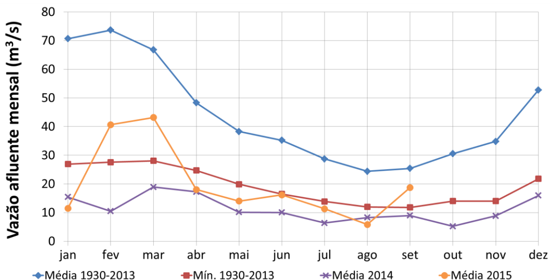
Figura 2. Vazão afluente (em m^3/s ) do Sistema Cantareira (Sistema Equivalente + Paiva Castro). A linha laranja refere-se à vazão média mensal até 23 de setembro de 2015 e a roxa à vazão média mensal de 2014. As linhas em azul e vermelho correspondem, respectivamente, às vazões médias mensais para o período 1930 – 2013 e aos mínimos absolutos da série histórica mensal no período 1930 – 2013.
