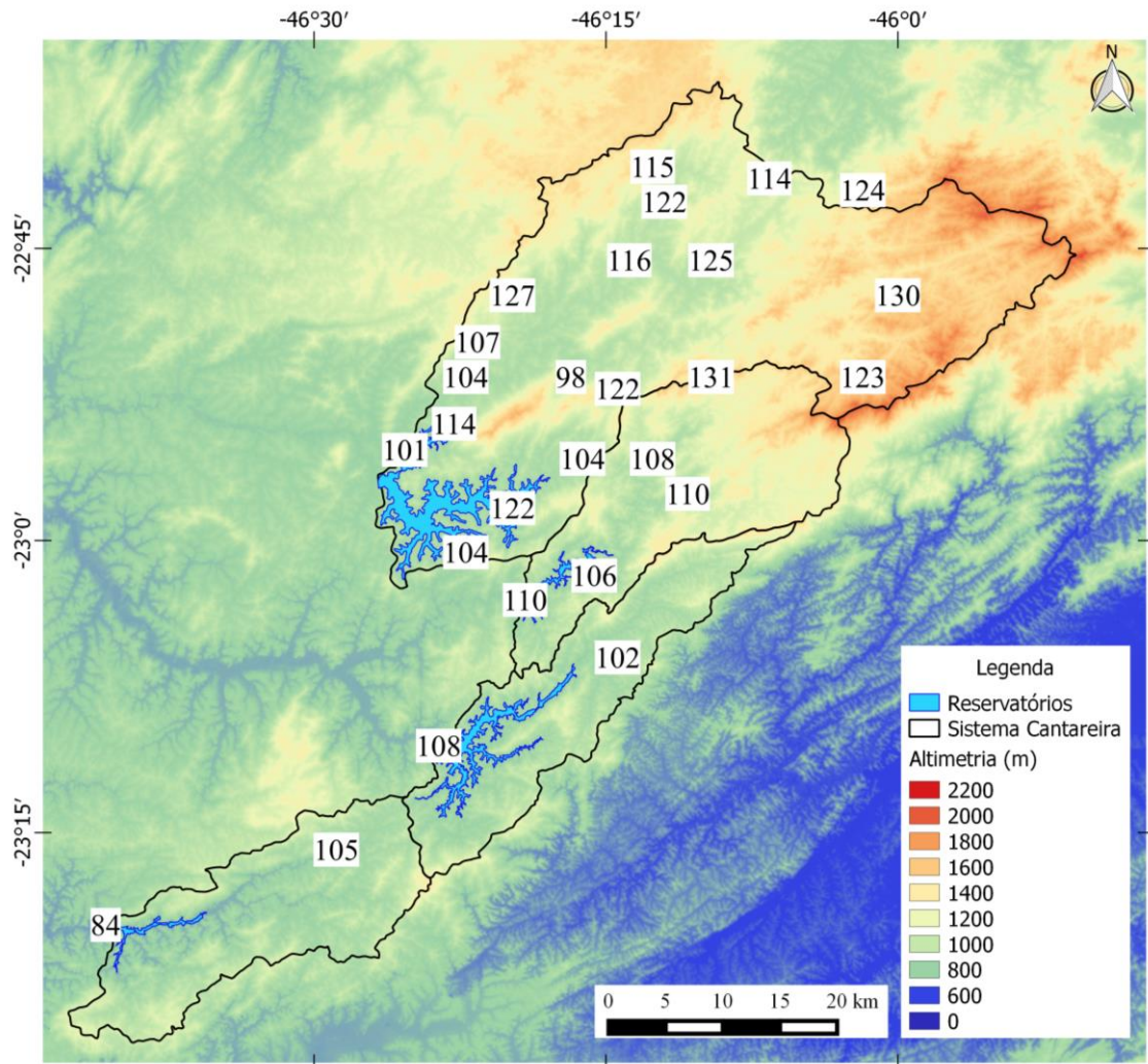
Figura 4. Precipitação observada acumulada (em mm) nos pluviômetros do CEMADEN e DAEE/SAISP nas sub-bacias de captação do Sistema Cantareira (contornos em preto). As cores representam alturas topográficas com relação ao nível do mar de acordo com a escala da direita.
