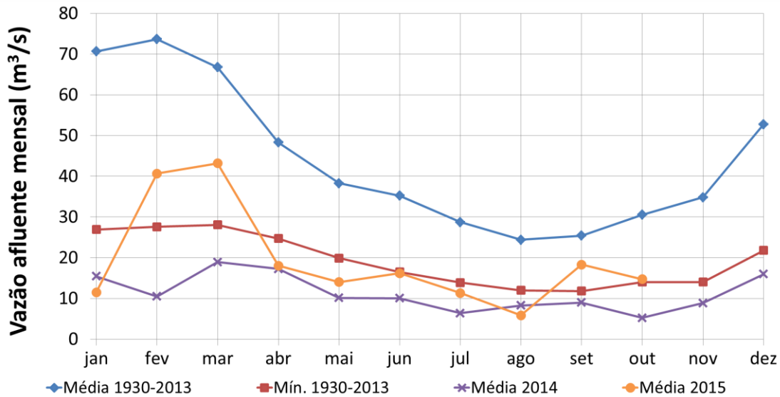
Figura 2. Vazão afluente (em m^3/s ) do Sistema Cantareira (Sistema Equivalente + Paiva Castro). A linha laranja refere-se à vazão média mensal até 29 de outubro de 2015 e a roxa à vazão média mensal de 2014. As linhas em azul e vermelho correspondem, respectivamente, às vazões médias mensais para o período 1930 – 2013 e aos mínimos absolutos da série histórica mensal no período 1930 – 2013.
