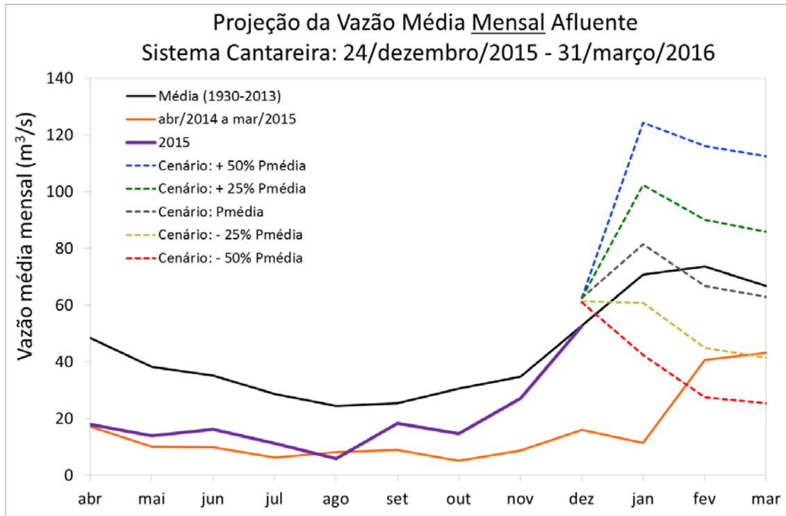
Figura 8. As linhas tracejadas apresentam cinco projeções de vazão média mensal afluente, em m^3/s , ao Sistema Cantareira (Sistema Equivalente + Paiva Castro) com a previsão do ETA/CPTEC/INPE para os próximos 7 dias e, na sequência, para os cenários: precipitação 50% abaixo da média climatológica (linha vermelha), 25% abaixo da média climatológica (linha amarela), na média climatológica (linha cinza), 25% acima da média climatológica (linha verde) e 50% acima da média climatológica (linha azul). O início das projeções corresponde à vazão média prevista para os próximos 7 dias e na sequência para a vazão projetada para cada cenário. A linha preta corresponde à vazão média mensal climatológica para o período 1930-2013, em laranja à vazão média mensal de abr/2014 a mar/2015 e em roxo de abril a 23 de dezembro de 2015.
