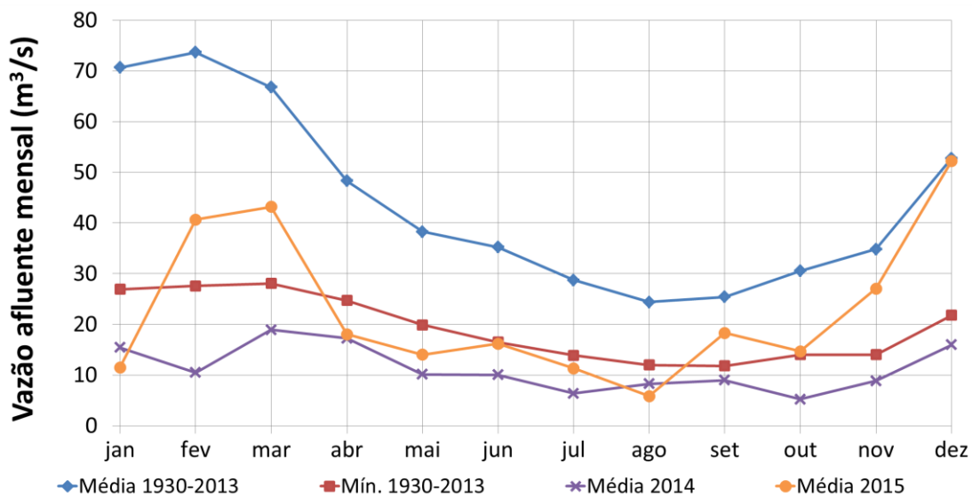
Figura 2. Vazão afluente (em m^3/s ) do Sistema Cantareira (Sistema Equivalente + Paiva Castro). A linha laranja refere-se à vazão média mensal até 30 de dezembro de 2015 e a roxa à vazão média mensal de 2014. As linhas em azul e vermelho correspondem, respectivamente, às vazões médias mensais para o período 1930 – 2013 e aos mínimos absolutos da série histórica mensal no período 1930 – 2013.
