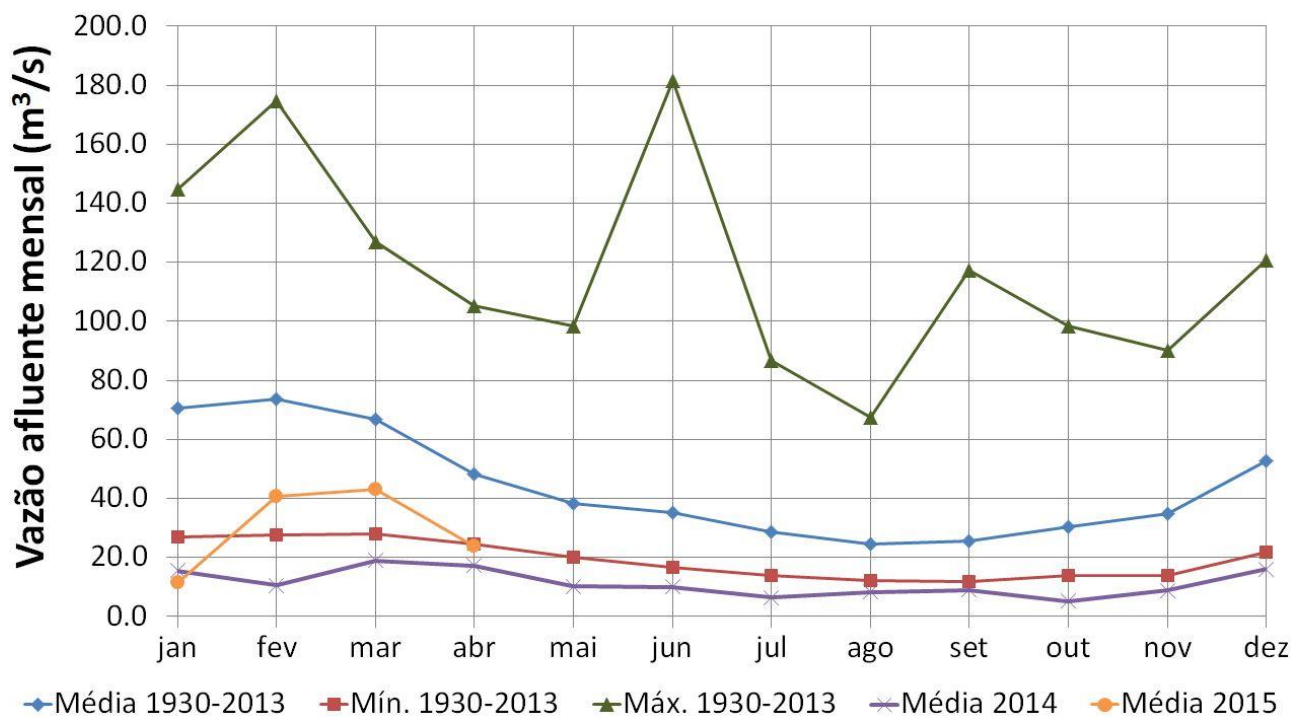
Figura 2. Vazão afluente (em m^3/s ) do Sistema Cantareira (Sistema Equivalente + Paiva Castro). A linha laranja refere-se à vazão média mensal até 08 de abril de 2015 e a roxa à vazão média mensal de 2014. A linha em azul corresponde às vazões médias mensais para o período 1930 – 2013. As linhas verde e vermelha referem-se, respectivamente, aos máximos e mínimos absolutos da série histórica mensal no período 1930 – 2013.
