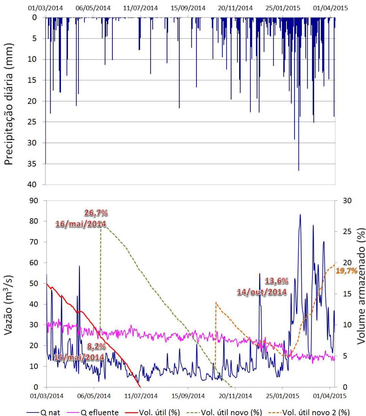
Figura 4. a) Precipitação média diária nas bacias do Sistema Cantareira (Dados do CEMADEN e DAEE) e b) Evolução da vazão afluyente ( Q_{nat} ) do Sistema Cantareira (linha azul), da vazão efluente ( Q_{efluente} = vazão para atendimento da demanda Região Metropolitana de São Paulo e Região de Campinas + vazão a jusante (linha magenta), e do volume útil (em porcentagem) do Sistema Cantareira (linha vermelha), do novo volume útil 1 (linha verde) e do novo volume útil 2 (linha laranja). As porcentagens correspondem ao volume útil de 982,0 \text{ hm}^3 (Fonte: SABESP – Situação dos mananciais e boletins diários da ANA – GTAG-Cantareira: situação dos reservatórios).
