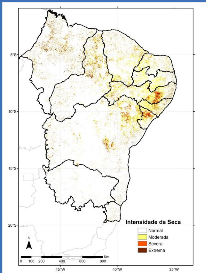
Figura 3 – Avaliação da intensidade da seca a partir da anomalia de VSWI para o mês de dezembro de 2016.
