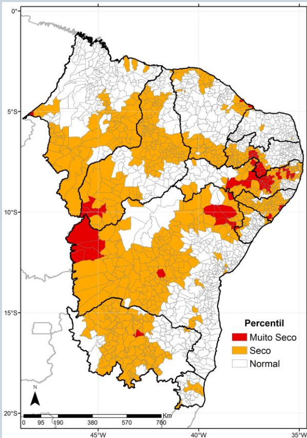
Figura 2 - Avaliação das condições de seca para os últimos 90 dias (03 de outubro a 31 de dezembro), de acordo com o cálculo dos percentis dos dados de precipitação.
