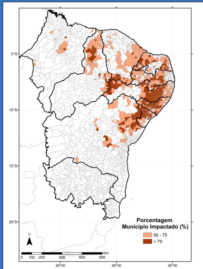
Figura 4 - Porcentagem do município impactado pela seca (impacto em áreas de pastagens e agrícolas) no mês de dezembro de 2016 de acordo com o índice VSWI.
