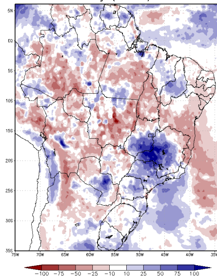
Figura 7 –(Esq.) Previsão de anomalia de precipitação no período 11 a 17 de dezembro de 2016, pelo modelo de previsão por conjuntos do NCEP/NOAA. (Dir.) Previsão de anomalia de precipitação no período 11 a 17 de dezembro de 2016, pelo modelo de previsão por conjuntos do CPTec/INPE.
