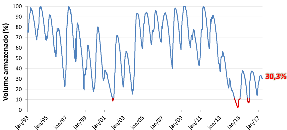
Figura 4. Evolução do volume armazenado do Aproveitamento Hidrelétrico Três Marias até 04 de junho de 2017 (em porcentagem do volume útil). (Fonte dos dados: Sistema de Acompanhamento de Reservatórios/ANA).
