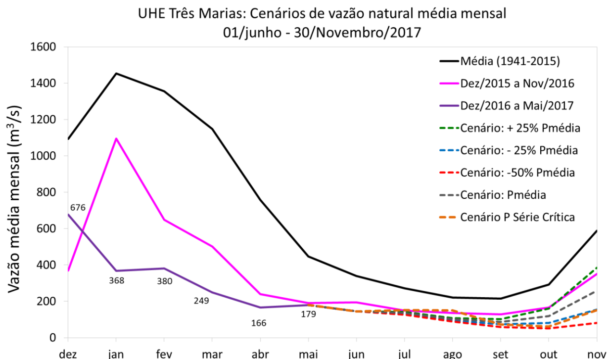
Figura 7. As linhas tracejadas apresentam cinco projeções de vazão média mensal afluyente, em m^3/s , ao Aproveitamento Hidrelétrico de Três Marias, um cenário de precipitação crítica (laranja) e os demais considerando a previsão do modelo ETA/CPTEC/INPE para os próximos 10 dias e, na sequência, os cenários: precipitação 50% abaixo da média climatológica (vermelha), 25% abaixo da média climatológica (azul), na média climatológica (cinza) e 25% acima da média climatológica (verde). A linha preta corresponde à vazão média mensal para o período 1941-2015; a linha magenta contínua, à vazão média mensal de dezembro de 2015 a novembro de 2016; e a linha roxa, de dezembro de 2016 a maio de 2017.
