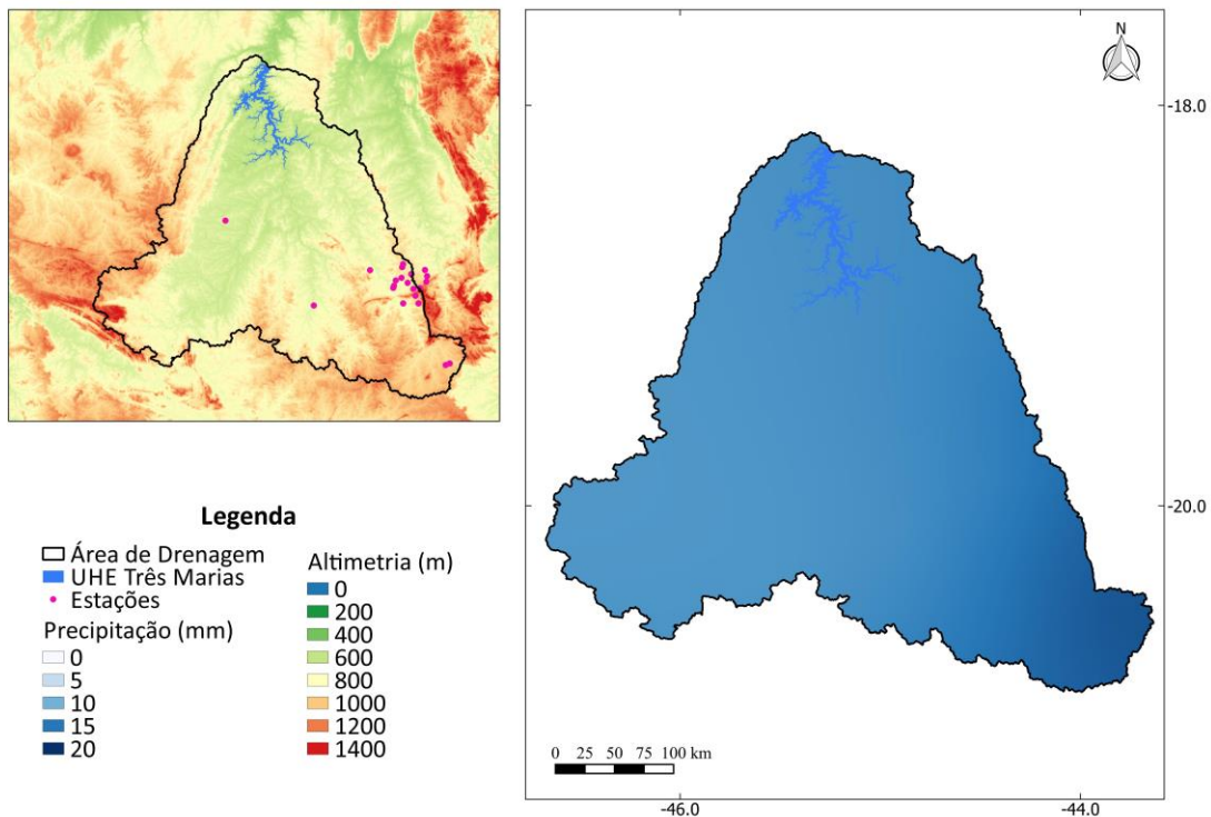
Figura 2. Precipitação observada (mm) na bacia de captação do Aproveitamento Hidrelétrico Três Marias delimitado pelo contorno em preto (esquerda) e localização dos pluviômetros ativos no mês de maio de 2018 (15 do CEMADEN e 11 do INMET) (direita). As cores, de acordo com a escala da legenda, representam respectivamente, a quantidade de precipitação obtida por interpolação dos dados dos pluviômetros e alturas topográficas com relação ao nível do mar.
