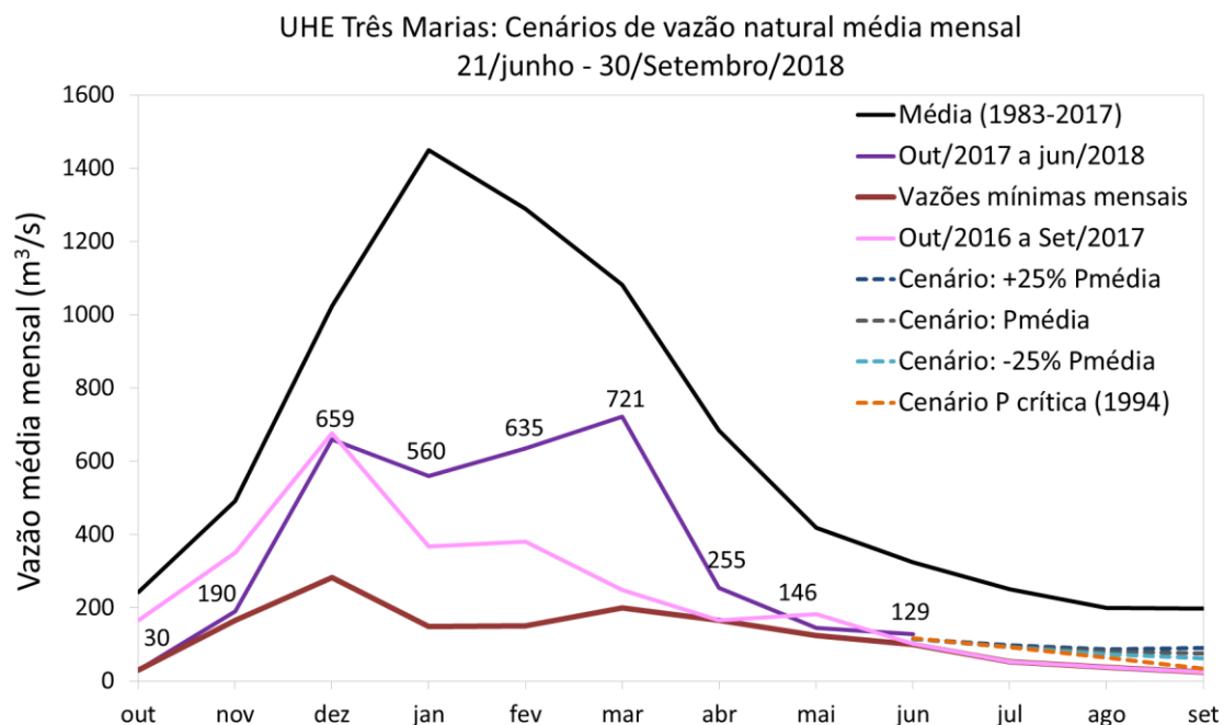
Figura 7. Cenários de vazão natural média mensal (em m 3 /s) para o aproveitamento Hidrelétrico de Três Marias (linhas tracejadas): precipitação 25% abaixo da média climatológica (azul claro); na média climatológica (cinza); 25% acima da média climatológica (azul escuro); e precipitação igual ao ocorrido em 1994 (laranja). As linhas espessas representam as vazões médias mensais observadas de acordo com a ONS: vazão média mensal para o período 1983-2017 (preto); vazão mínima média mensal para o período 1983-2017 (marrom); vazão média mensal de outubro de 2016 a setembro de 2017 (rosa); e vazão média mensal de outubro de 2017 a junho de 2018 (roxo).
