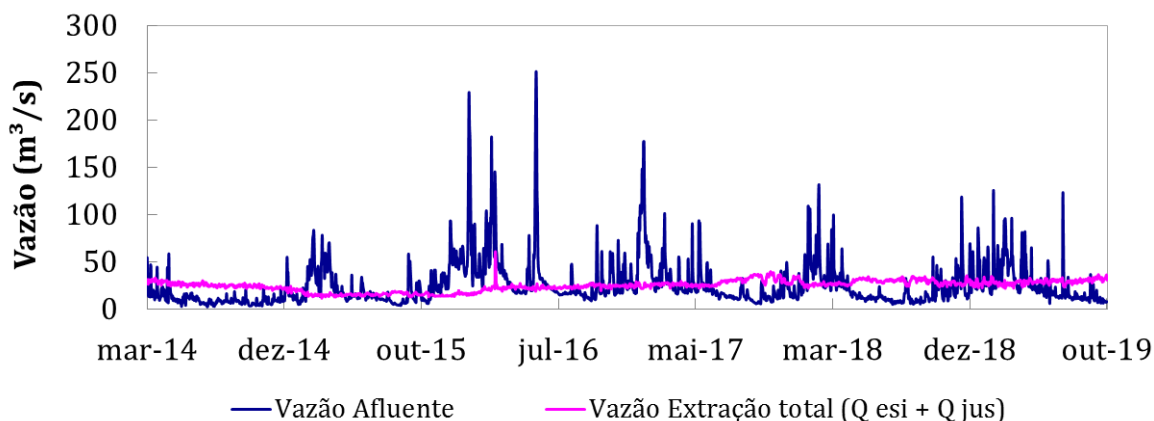
Figura 4. Evolução da vazão afluente (em m 3 /s) do Sistema Cantareira (linha azul) e da vazão de extração total: vazão para atendimento da demanda da Região Metropolitana de São Paulo - Q esi - somada à vazão a jusante para a bacia dos rios Piracicaba, Capivari e Jaguari - Q jus (linha magenta). Fonte dos dados: SABESP.
