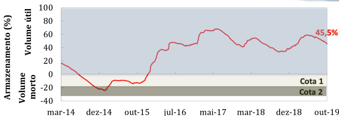
Figura 5. Evolução do nível de armazenamento (%) do Sistema Cantareira. Área em cinza corresponde ao volume útil do reservatório (982 hm 3 ), em marrom claro à primeira cota do volume morto (182,5 hm 3 ) e em marrom escuro à segunda cota do volume morto (105 hm 3 ). Fonte dos dados: SABESP.
